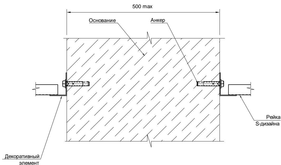
Разрез А-А
