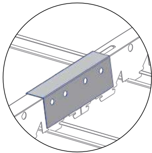
6. Соед. элемент для гребенки
