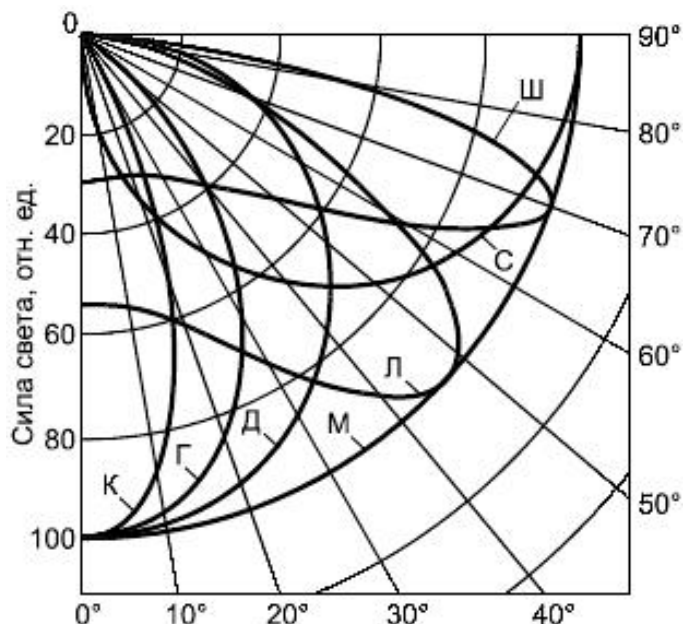
Рисунок 1 - Типы кривых силы света
