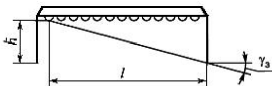
д — для светильников со светодиодами
