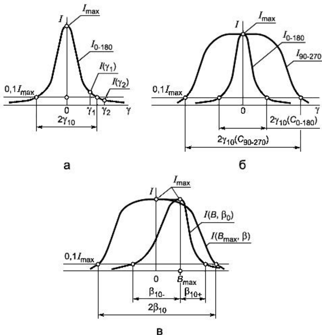
Рисунок 4 - Определение углов рассеяния прожектора
