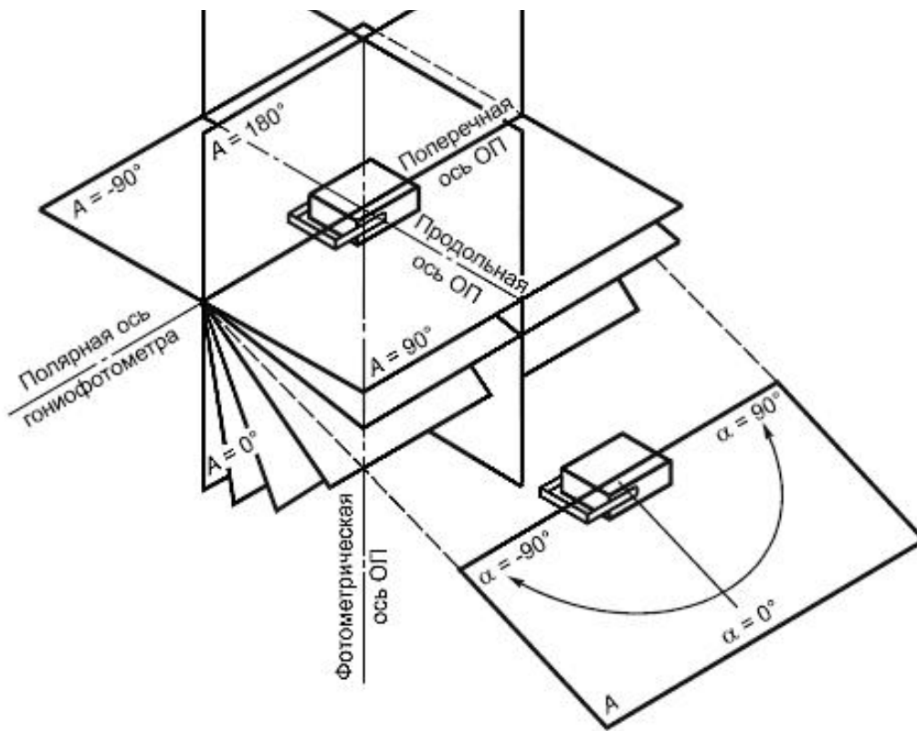
в – система фотометрирования A, \alpha
