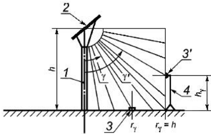
а - вид сбоку
