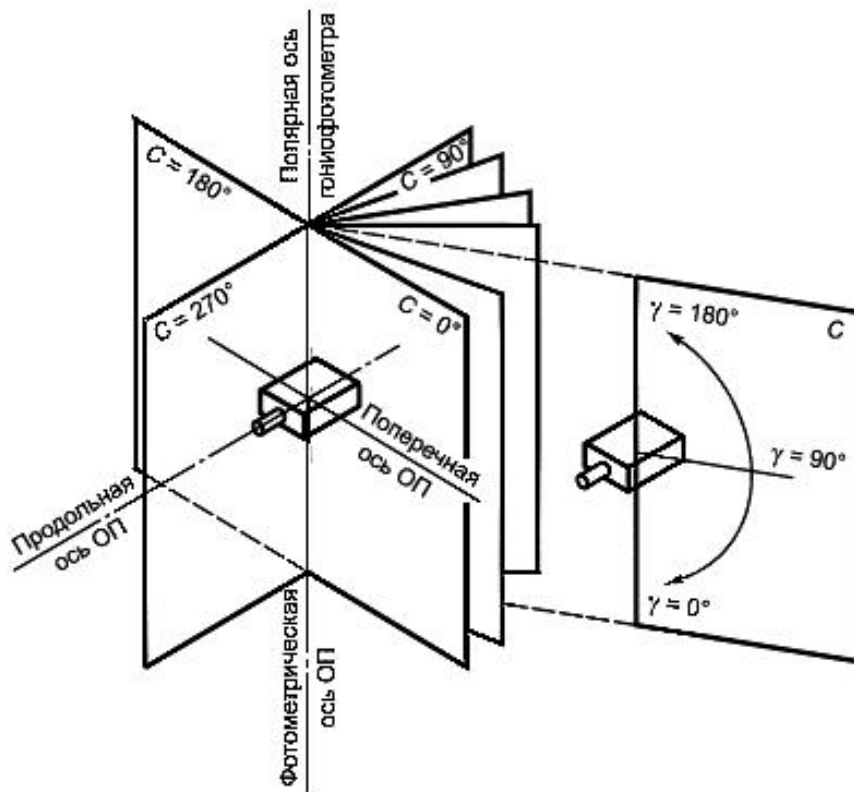
а – система фотометрирования C, \gamma
