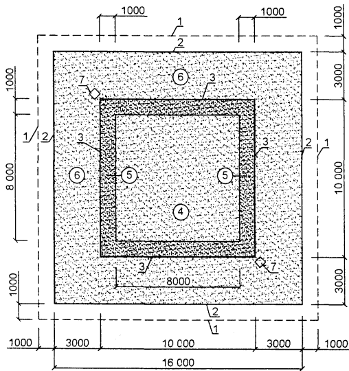
СХЕМА ПЛАНА АРЕНЫ ДЛЯ СОРЕВНОВАНИЙ ПО ДЗЮДО
