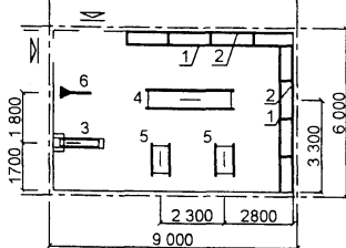
Зал 9×6 м для занятий с использованием тренажерной техники
