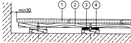
Схема 3. Пол на амортизирующей подложке
