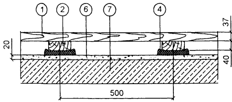
Схема 2. Пол по двойным лагам
