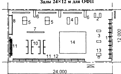
Залы 24×12 м для ОФП
