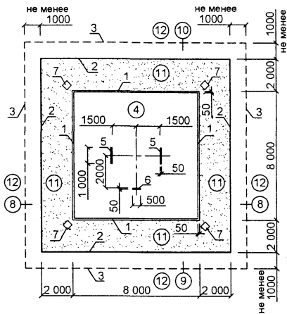
СХЕМА ПЛАНА АРЕНЫ ДЛЯ СОРЕВНОВАНИЙ ПО ДЗЮДО
