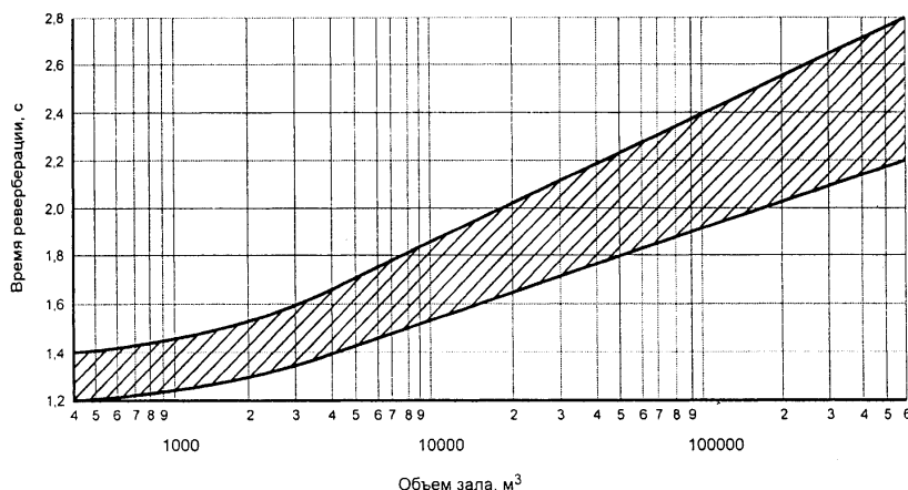
Рисунок 7.1 — График времени реверберации
