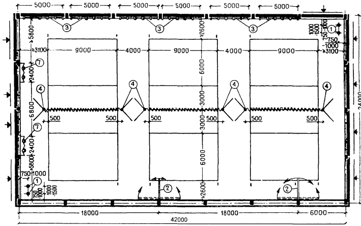
ЗАЛ ДЛЯ ВОЛЕЙБОЛА
