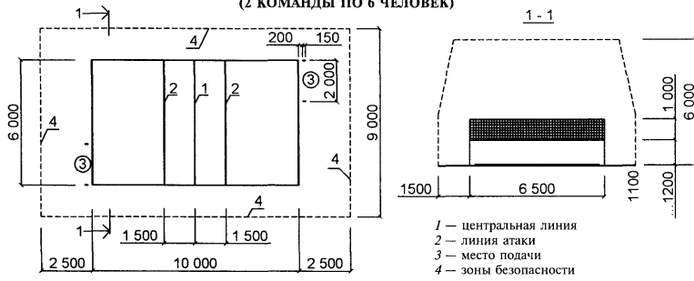
Б. ПЛОЩАДКА И ЗАЛ ДЛЯ БАСКЕТБОЛА СИДЯ (2 КОМАНДЫ ПО 5 ЧЕЛОВЕК)
