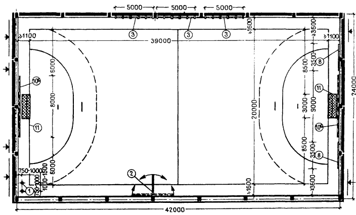
ЗАЛ ДЛЯ ГАНДБОЛА
