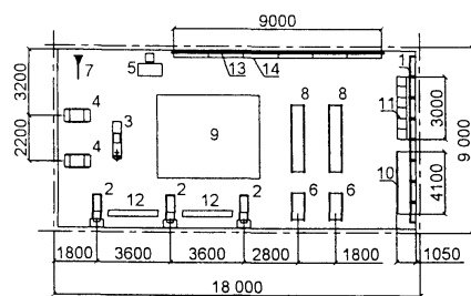
ОБОРУДОВАНИЕ ЗАЛА 18×9 м
