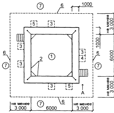
СХЕМА ПЛАНА АРЕНЫ ДЛЯ СОРЕВНОВАНИЙ ПО БОКСУ
