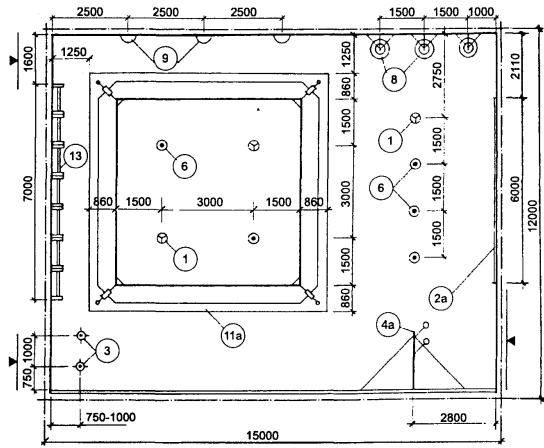
ПЛАН ЗАЛА 15×12 м ДЛЯ УЧЕБНО-ТРЕНИРОВОЧНЫХ ЗАНЯТИЙ
