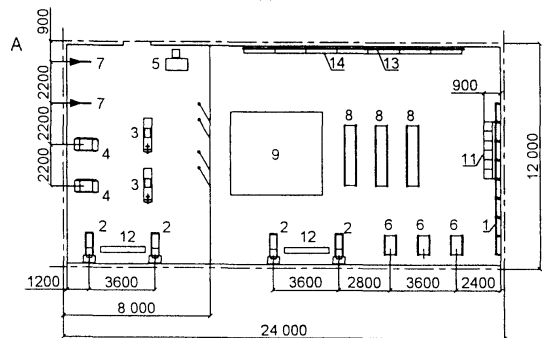
ВАРИАНТЫ ОБОРУДОВАНИЯ ЗАЛА 24×12 м
