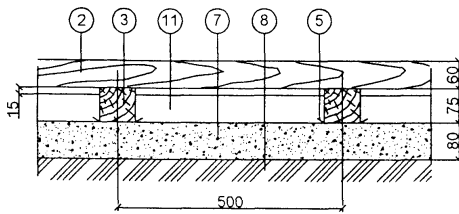
Схема 4. Брусчатый пол по лагам на перекрытии
