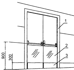
Схема входной двери в зал
