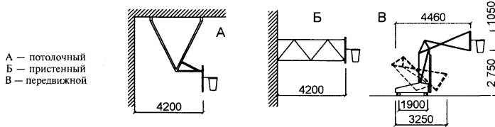
РЕКОМЕНДУЕМЫЕ КОНСТРУКЦИИ БАСКЕТБОЛЬНЫХ ЩИТОВ
