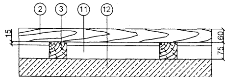
Схема 4. Брусчатый пол по лагам на перекрытии
