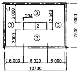
ЗАЛ ДЛЯ ИГРЫ В ШОУ-ДАУН
