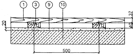
Схема 3. Брусчатый пол по лагам на грунте
