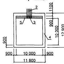
Зал с уменьшенной полосой ориентации
