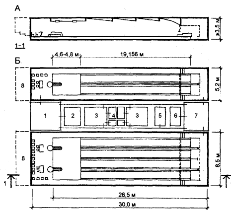
Планировочная схема кегельбана
