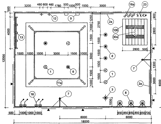
ПЛАН ЗАЛА 18×12 м ДЛЯ УЧЕБНО-ТРЕНИРОВОЧНЫХ ЗАНЯТИЙ
