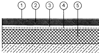
Схема 3. Пол с синтетическим покрытием заливного типа
