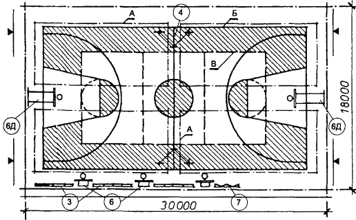
А. Зал 30×18 м для: бадминтона (А), баскетбола (Б), волейбола (В)
