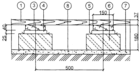
Схема 2. Дощатый пол по лагам на перекрытии
