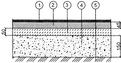
Схема 2. Пол по перекрытию
