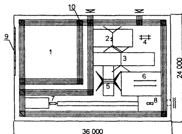
ЗАЛ 24×36 м ДЛЯ СПОРТИВНОЙ ГИМНАСТИКИ
