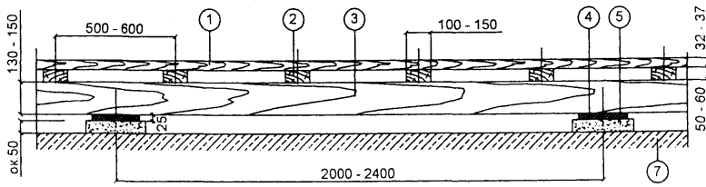
Схема 2. Пол по двойным лагам
