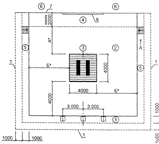
СХЕМА ПЛАНЫ АРЕНЫ ДЛЯ СОРЕВНОВАНИЙ ПО ТЯЖЕЛОЙ АТЛЕТИКЕ
